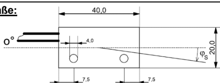
Bezugsebene für den angegebenen Schaltwinkel ist die Gehäuse-unterseite.
